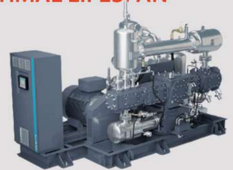
CO2 COMPRESSOR
